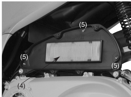
(4) Filtro aria (5) Viti interne
