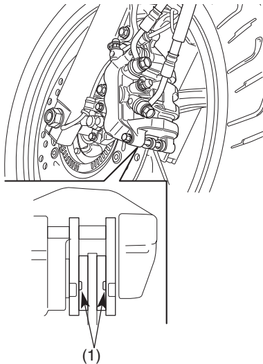
(1) Segno di indicazione usura
