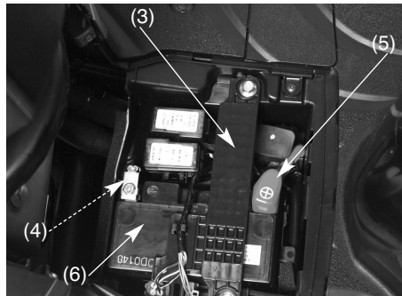
(3) Staffa batteria (4) Cavo terminale negativo (-) (5) Cavo terminale positivo (+) (6) Batteria
