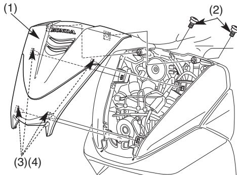
(1) Scudo frontale (2) Viti superiori
