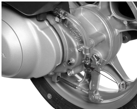
(1) Tappo di tubo sfiato carter
