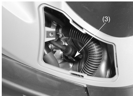
(3) Pipetta candela
